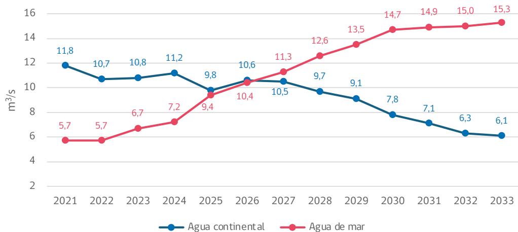
Figura 14: Proyección demanda de agua en la minería del cobre.
