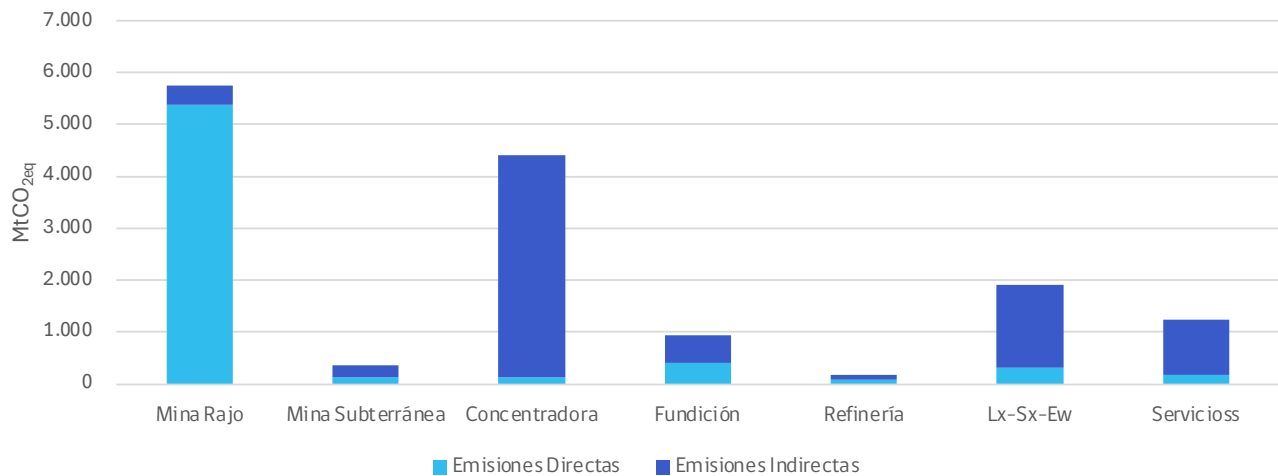
Figura 17: Emisiones de Alcance 1 y Alcance 2 por proceso.
