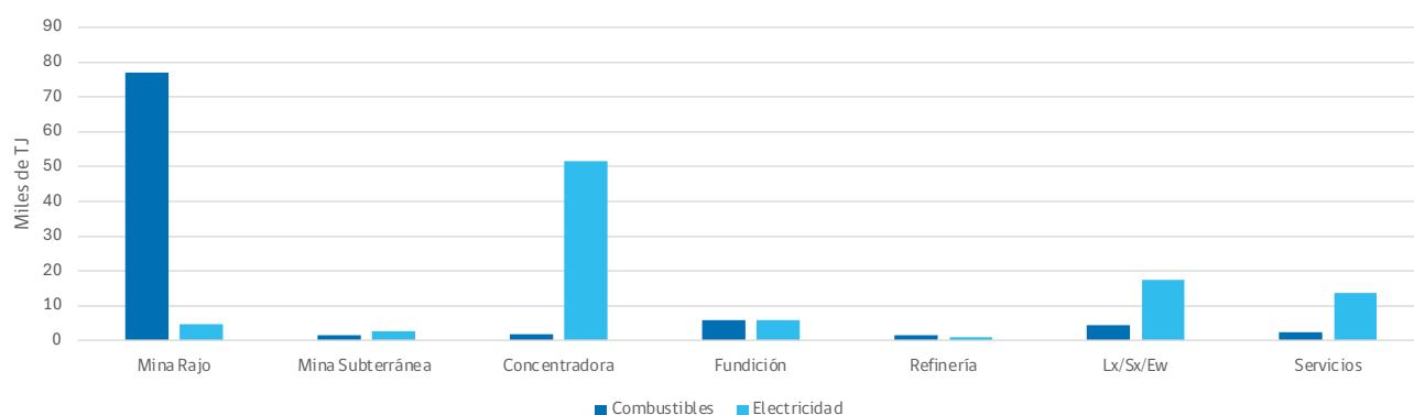
Figura 10: Consumo de electricidad y combustible por actividad en la minería del cobre al 2023.
