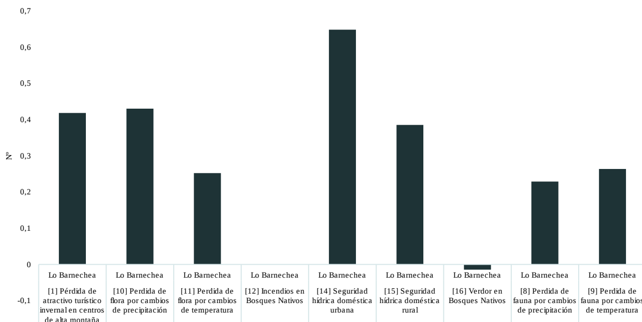
Gráfico 1: Análisis de riesgos en las comunas clasificadas en la tipología montaña. Fuente: Elaboración propia con información contenida en la Plataforma ARClím.
