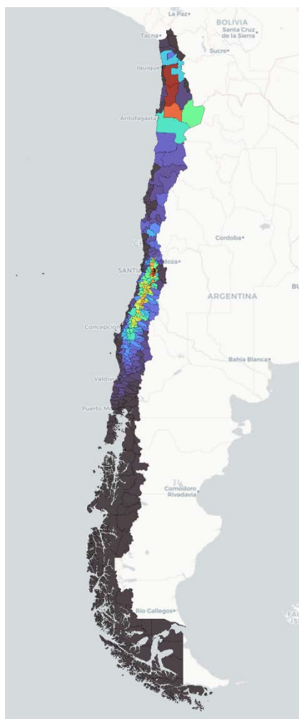
Figura 20. Variación de los eventos de olas de calor (>3 días con temperaturas >30°C) en el territorio nacional. Fuente: ARCLim, MMA (2020).
