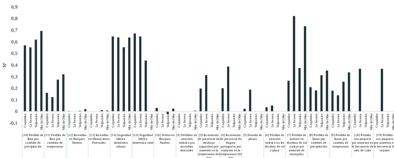
Gráfico 3: Análisis de riesgos en las comunas clasificadas en la tipología Urbano y litoral. Fuente: Elaboración propia con información contenida en la Plataforma ARCLim.
