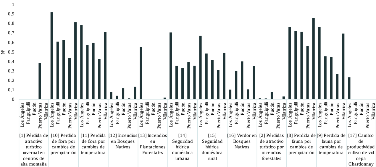
Gráfico 4: Análisis de riesgos en las comunas clasificadas en la tipología Lacustre y fluvial. Fuente: Elaboración propia con información contenida en la Plataforma ARClím.
