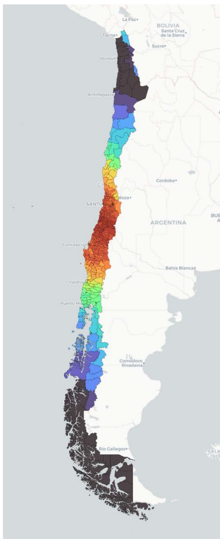
Figura 22 Variación de la frecuencia de sequías en el territorio nacional. Fuente: ACLlím, MMA (2020).
