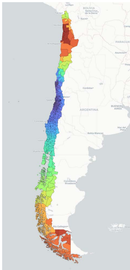
Figura 21 Variación de las precipitaciones anuales en el territorio nacional. Fuente: ARClím, MMA (2020).
