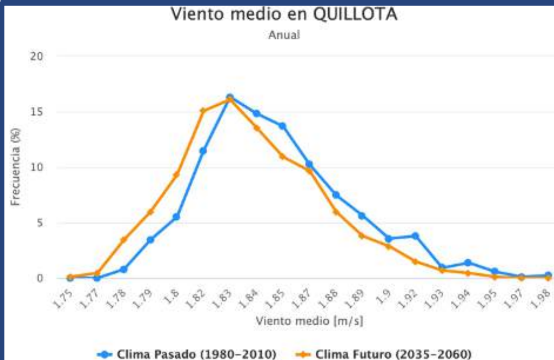
IMAGEN N° XXXX: DISTRIBUCIÓN DE FRECUENCIA VIENTO MEDIO EN LA COMUNA DE QUILLOTA
