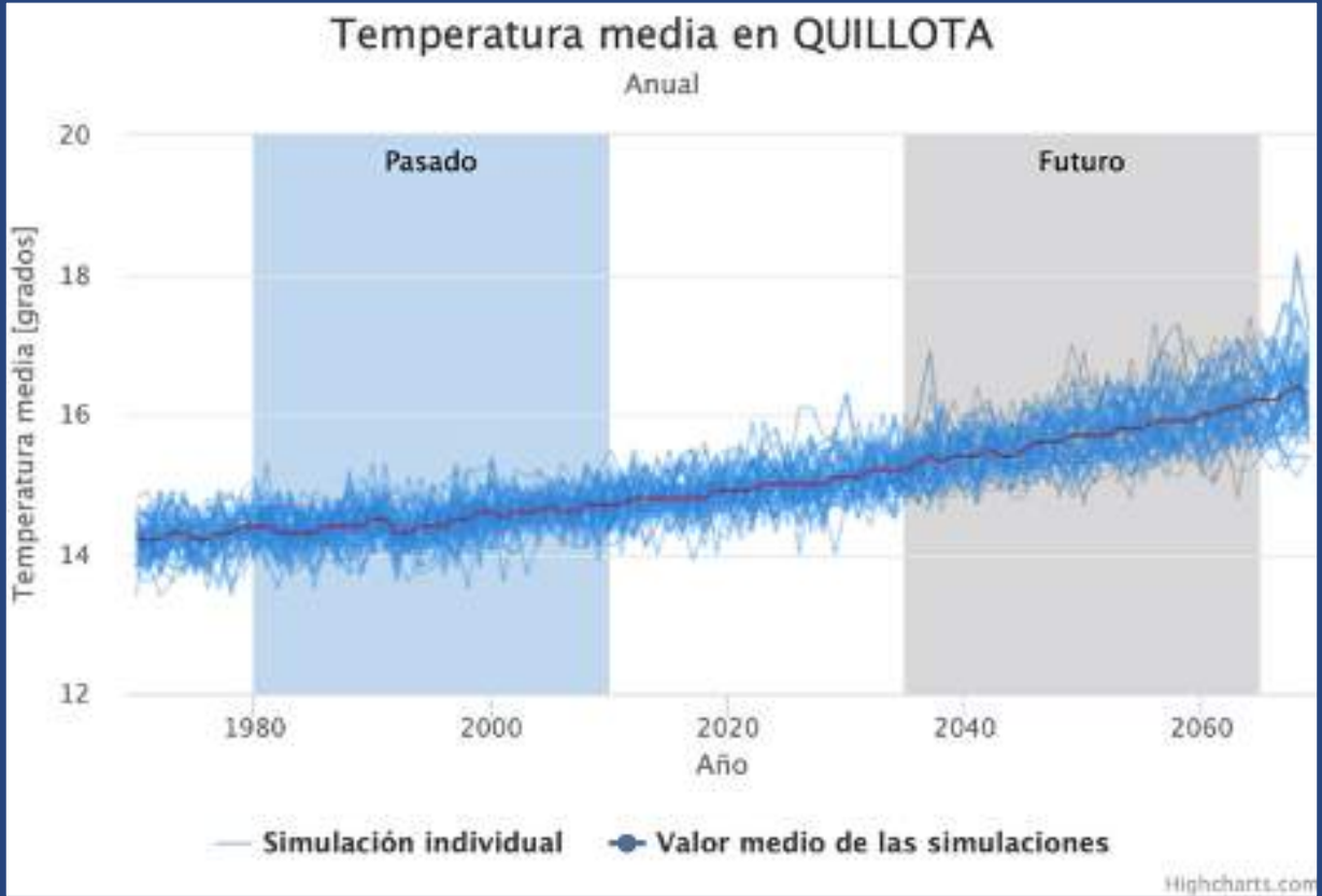
IMAGEN N° XXXX: SERIE DE TIEMPO TEMPERATURA MEDIA EN QUILLOTA
