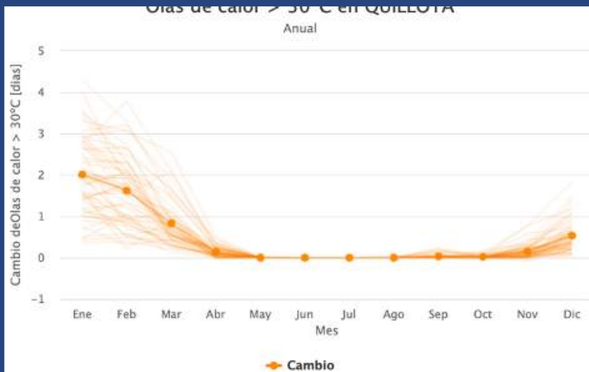
IMAGEN N° XXXX: CICLO ANUAL CAMBIO OLA DE CALOR > 30°C EN QUILLOTA
