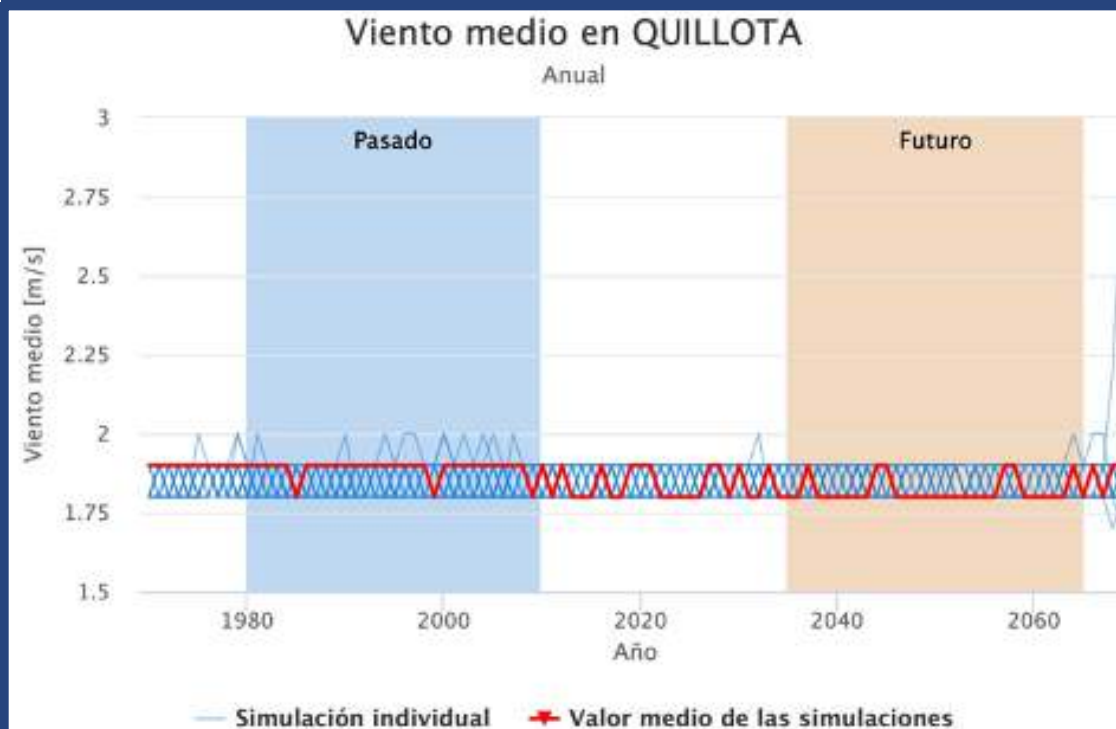
IMAGEN N° XXXX: SERIE DE TIEMPO VIENTO MEDIO EN LA COMUNA DE QUILLOTA
