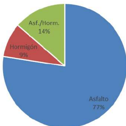
Figura 46: Longitud de dobles calzadas Región Metropolitana por capa de rodadura - diciembre 2021
